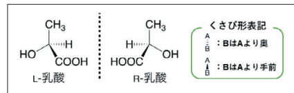
図6 乳酸の鏡像異性体
