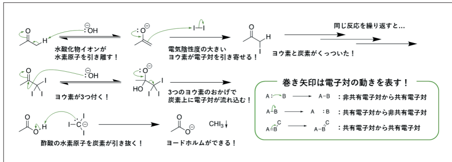
図5 ヨードホルム反応の機構
