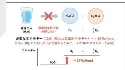
図4 エネルギーから説明する水の分解
