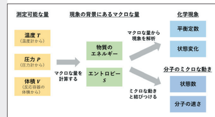
図3 測定可能な量からマクロな熱力学量を捉える
