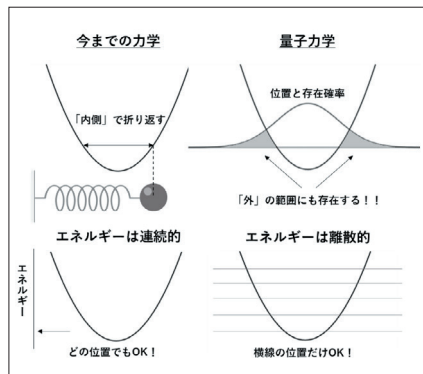
図1 今までの力学と量子力学の違い
